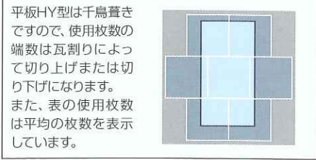
和瓦用下地ユニット0404タイプ
