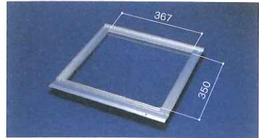
和瓦・平板瓦用下地ユニット0408タイプ
